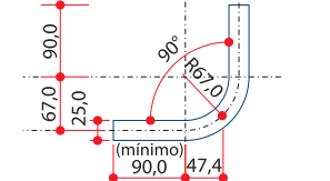
TUBO DE 1"(externo) em chapa 2,25mm
