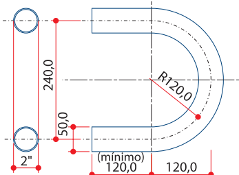
TUBO DE 2"(externo) em chapa 2,25mm
