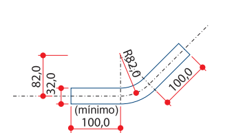
TUBO DE 1.1/4"(externo) em chapa 2,25mm
