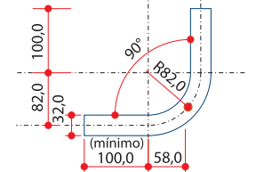
TUBO DE 1.1/4"(externo) em chapa 2,25mm
