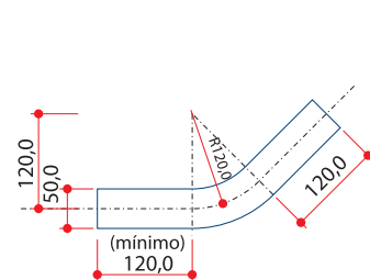
TUBO DE 2"(externo) em chapa 2,25mm
