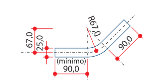
TUBO DE 1"(externo) em chapa 2,25mm
