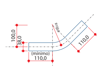
TUBO DE 1.1/2"(externo) em chapa 2,25mm
