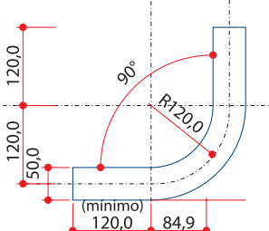
TUBO DE 2"(externo) em chapa 2,25mm
