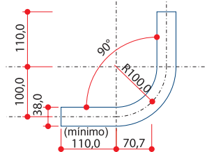
TUBO DE 1.1/2"(externo) em chapa 2,25mm
